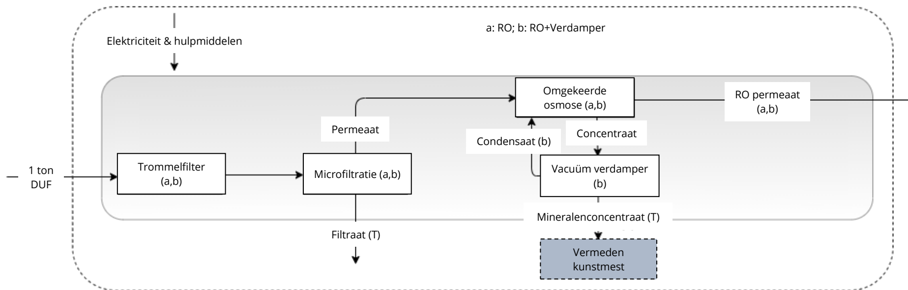
Figuur 3: Scenario 3 – RO (+ Verdamer).
