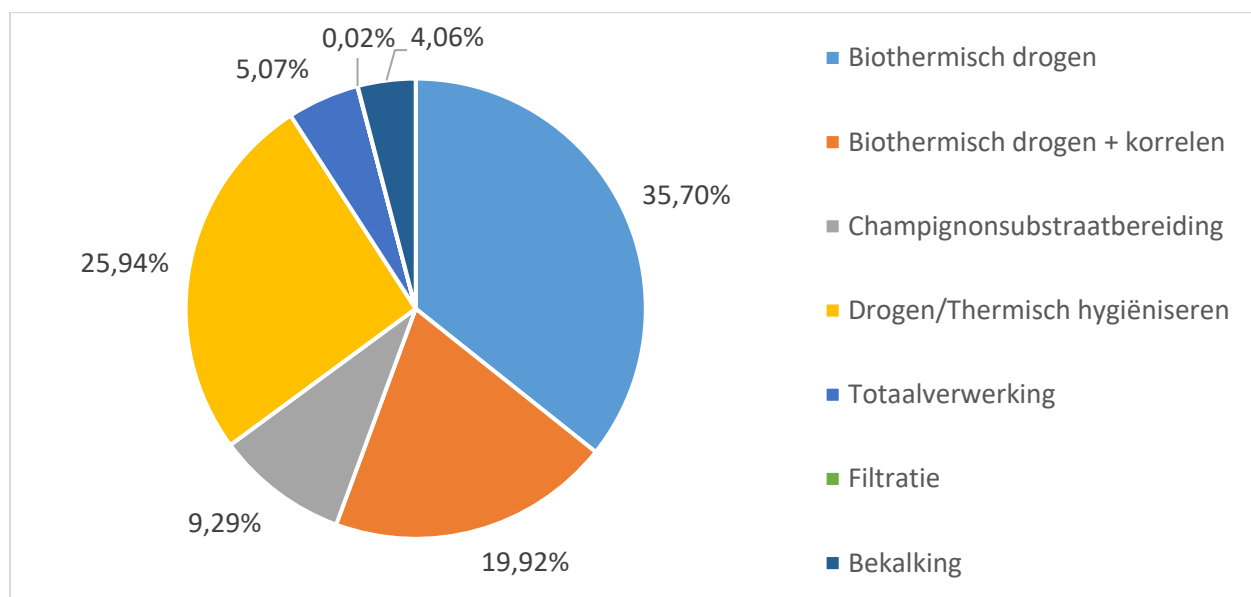
Figuur 14: Procentueel aandeel van de hoeveelheid P_2O_5 die via de verschillende primaire technieken wordt verwerkt (excl. export). Biologie en Biologie met constructed wetlands vormen in de tekst samen de categorie 'Biologische verwerking' en Biothermisch drogen en Biothermisch drogen + Korrelen vormen in de tekst samen de categorie 'Biothermisch drogen'.
