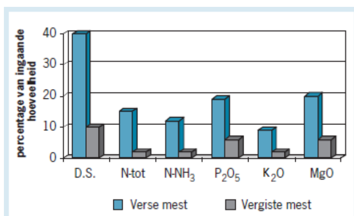
Figuur 6 Scheidingsrendement voor droge stof en mineralen van de vijzelpers bij scheiding verse varkensmengmest en vergiste varkensmengmest (de Buissonjé & Smolders, 2002). DS: Droge Stof.
